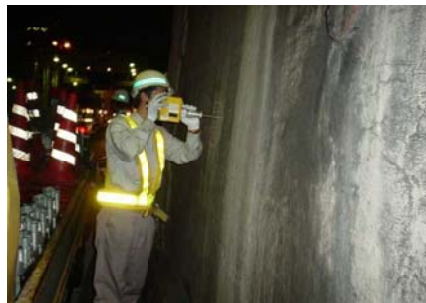
シュミットハンマー試験
